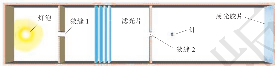
图 2-21 泰勒的光的衍射实验
