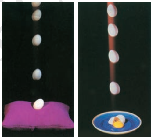
图 1-3 下落的鸡蛋
