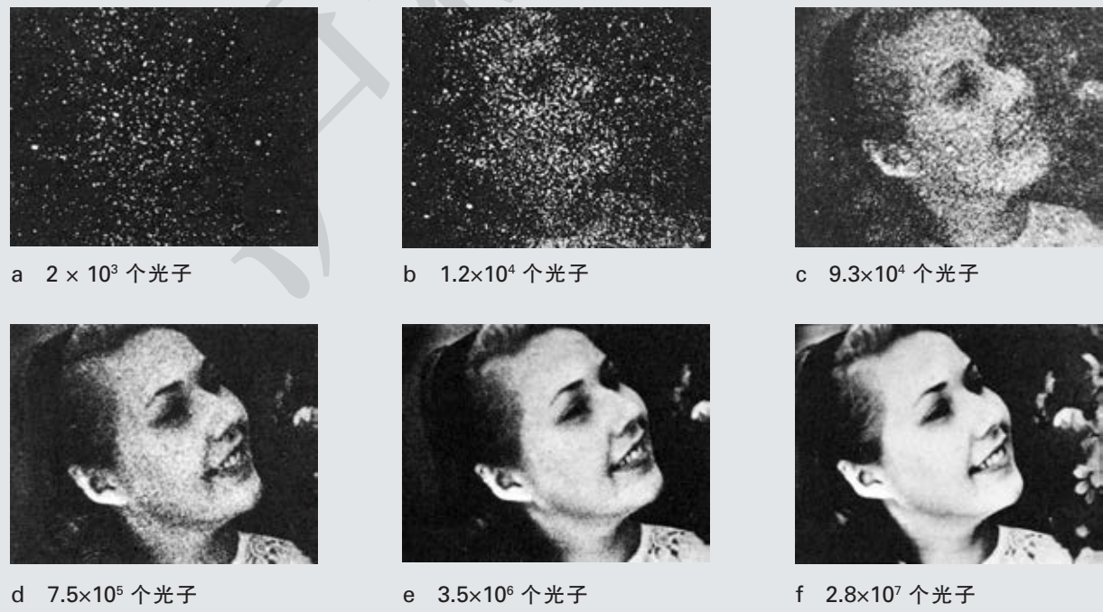
图 2-22 用不同曝光量洗印的照片
