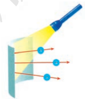
图 2-9 光电效应现象
