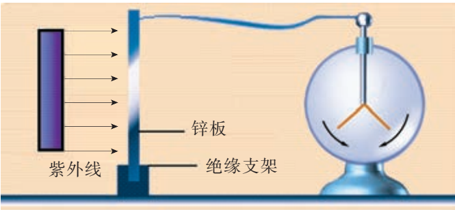
图 2-10 光电效应实验
