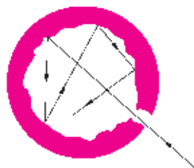
图 2-7 近似的黑体
