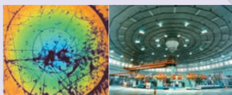
图 4-1 云雾中的粒子径迹
