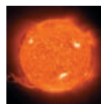
图 5-15 太阳释放的能量是通过热核反应产生的
