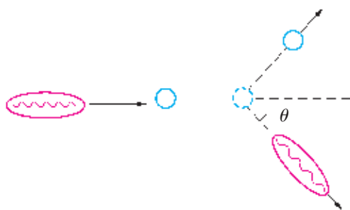
图 2-16 康普顿效应中的 光子和电子的碰撞
