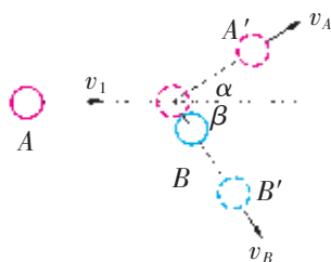
图 1-31 两球的斜碰
