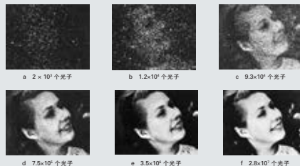
图 2-22 用不同曝光量拍摄的照片
