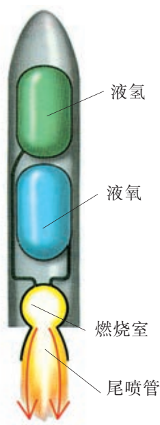
图 1-27 火箭
