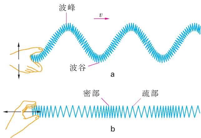
图 2-8 弹簧上的横波与纵波
