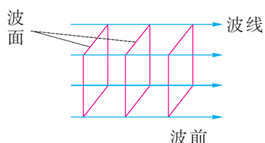
图 2-20 平面波
