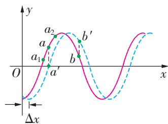
图 2-17 波的传播示意图
