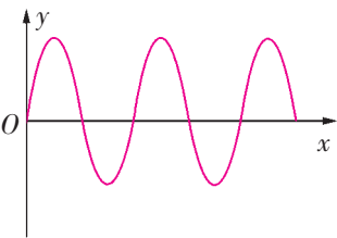
图 2-10 波的图像
