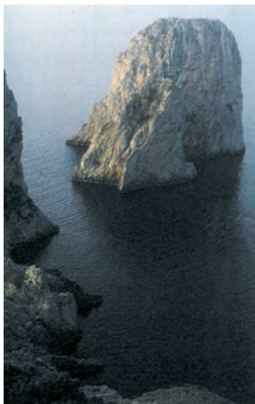
图 2-36 水波绕过山
