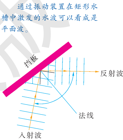
图 2-23 水波的反射规律
