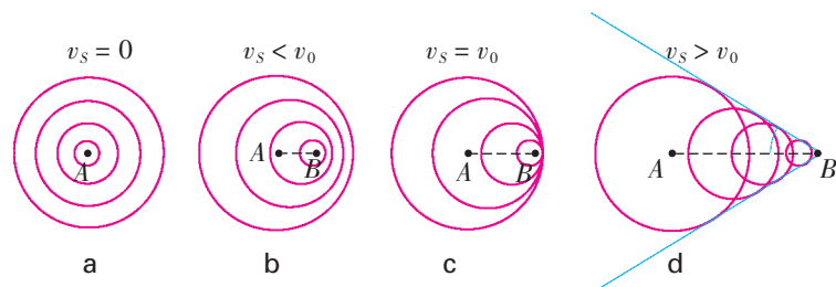
图 2-46 冲击波的形成过程
