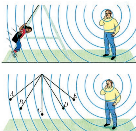
图 2-43 体验哨声的变化
