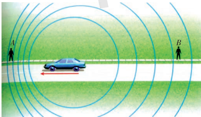
图 2-44 产生多普勒效应的原理示意图
