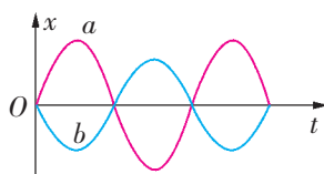
图 1-25 两个反相振动的图像
