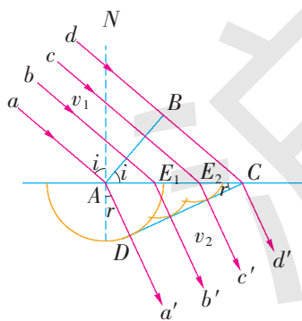
图 2-27 波的折射
