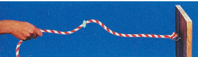
图 2-6 绳中的横波
