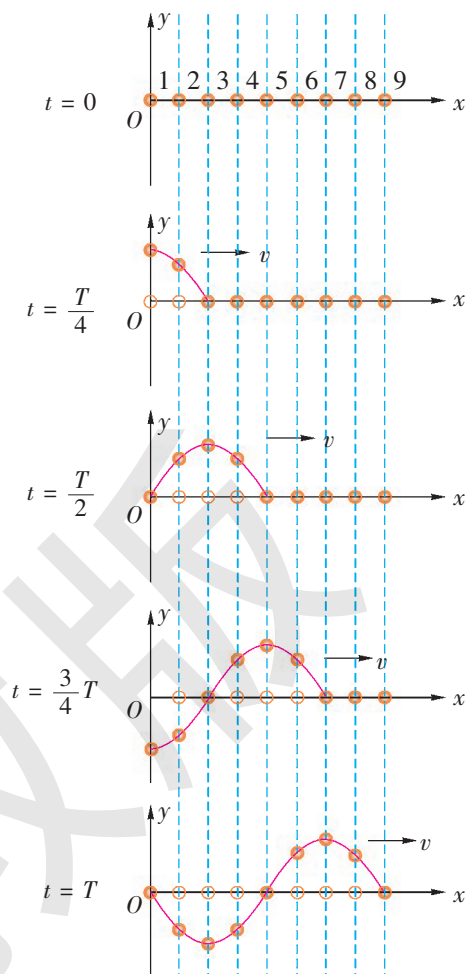
图 2-7 探究机械波的形成
