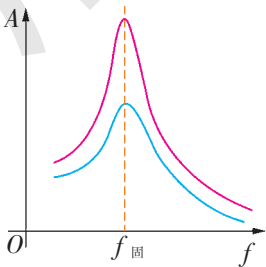
图 1-35 共振图像
