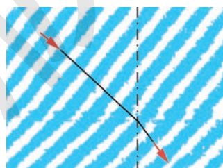
图 2-26 水波折射图样
