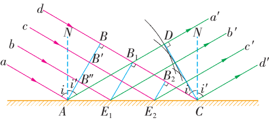
图 2-24 波的反射
