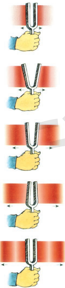
图 2-9 声波是纵波
