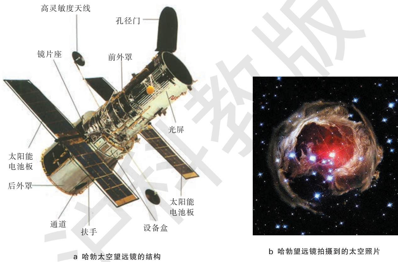
图 1-38 哈勃太空望远镜
