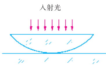
图 2-29 用牛顿环检验透镜质量示意图
