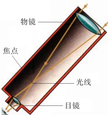
图 1-31 开普勒望远镜结构示意图
