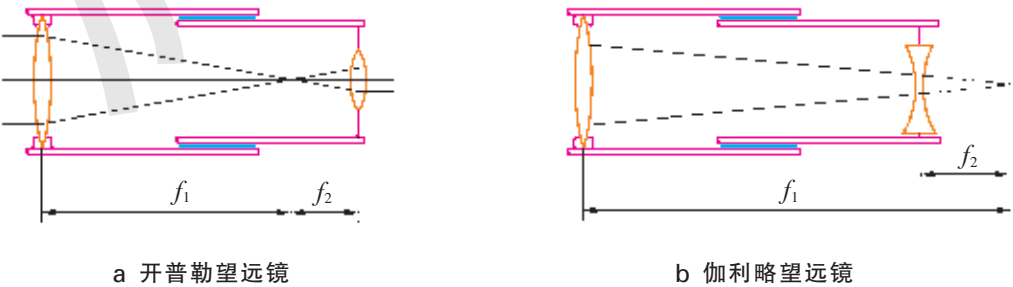
图 1-39 望远镜的结构
