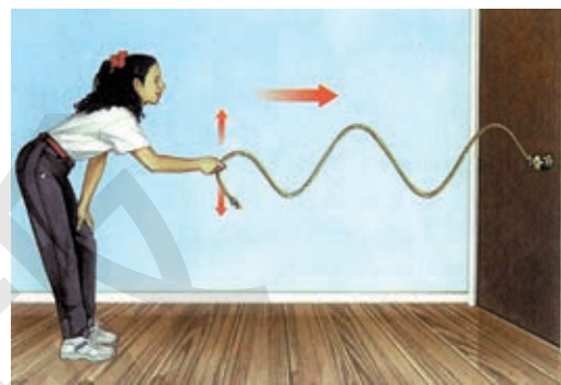
图 2-4 绳子上的横波
