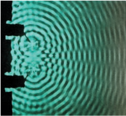
图 2-21 水波的干涉
