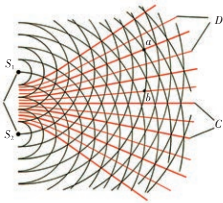
图 2-22 波的干涉示意图
