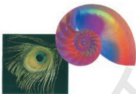
图 2-36 孔雀羽毛和珍珠母产生的衍射和干涉现象
