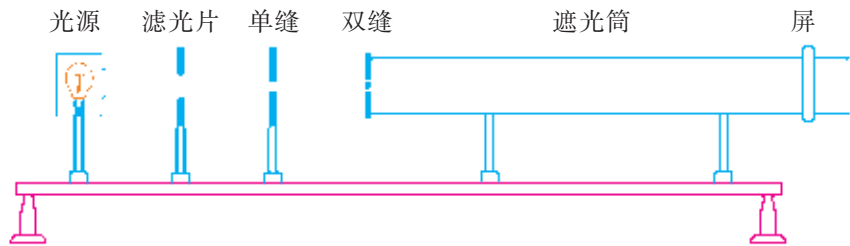
图 2-23 双缝干涉仪
