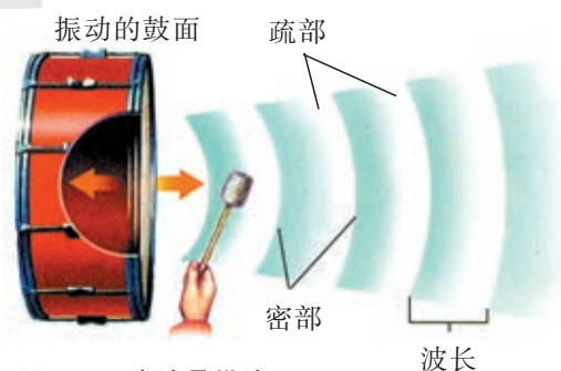
图 2-5 声波是纵波
