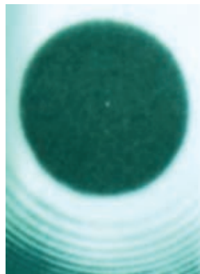
图 2-37 泊松亮斑
