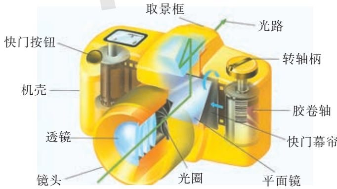
图 1-3 普通照相机的基本结构
