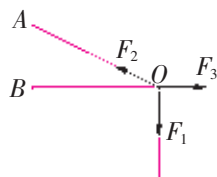
图 2-10 塔吊吊臂端点 O 的受力图
