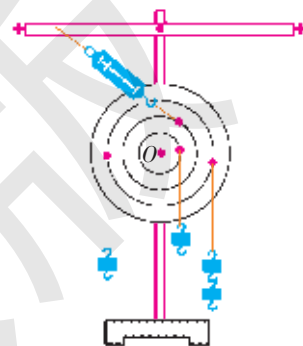
图 2-18 探究有固定转动轴物体的平衡条件
