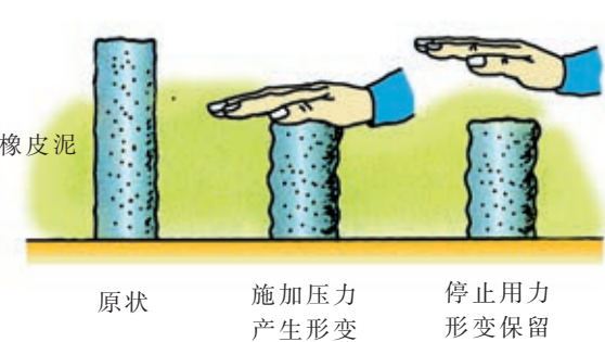
图 1-9 范性形变
