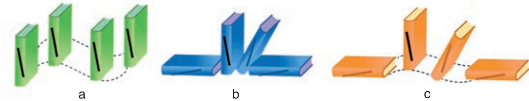
图 2-5 平动与转动
