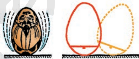
图 2-35 不倒翁
