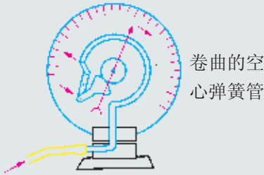
图 1-11 气压表
