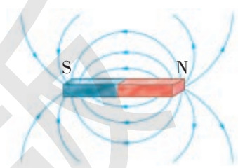
条形磁铁的磁感线
