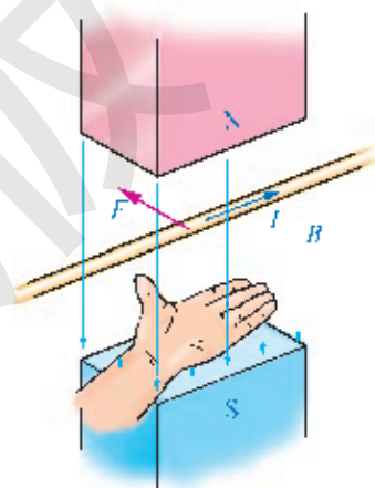
图 2-17 左手定则
