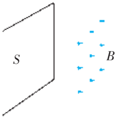
图 2-22 磁通量的意义
