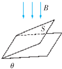
图 2-24 如何计算磁通量
