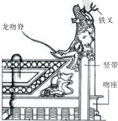
图 1-15 我国许多古建筑屋顶上的龙须也是一种很好的避雷装置
