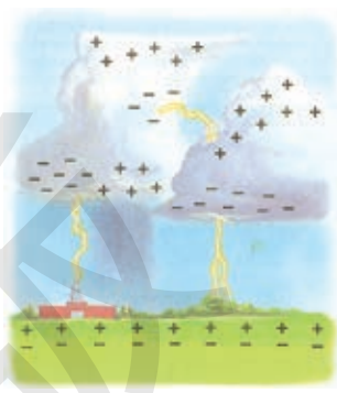
图 1-2 云层积聚电荷
