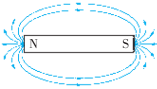
图 2-20 条形磁铁的磁感线
