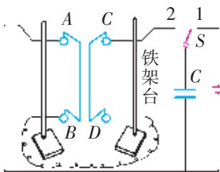
图 2-14 通电直导线的相互作用
