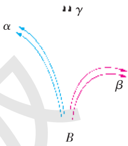
图 2-49 三种射线
