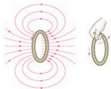
图2-7 环形电流产生的磁场
