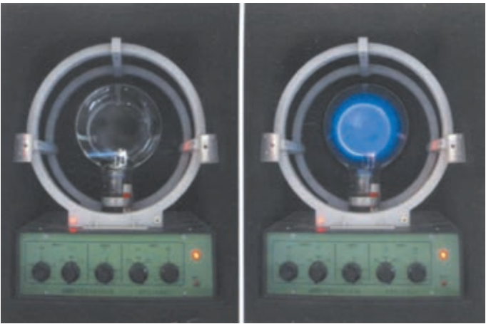
a 无磁场时电子束的径迹 b 有磁场时电子束的径迹
