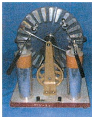
图 1-3 起电机
