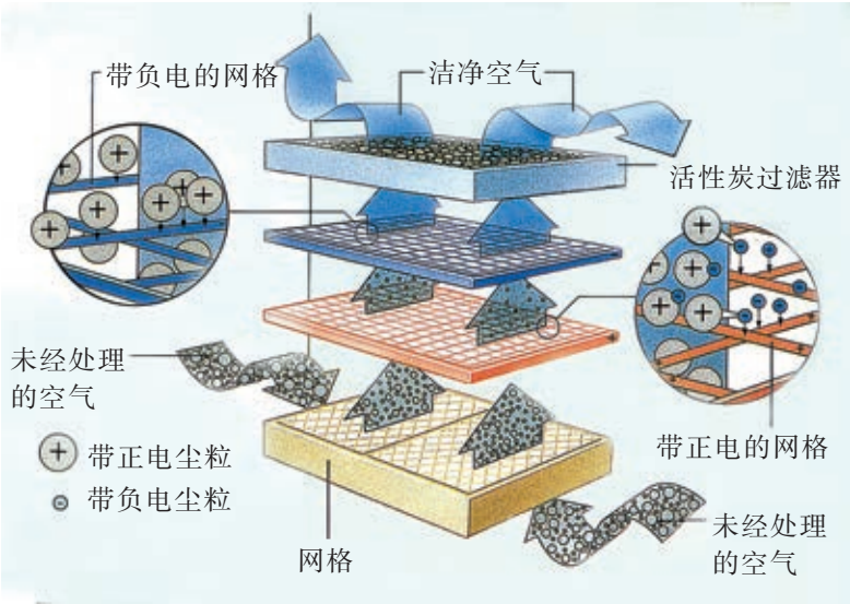
空气通过带电的网格,空气中带正电的微粒被吸附,再经活性炭过滤器过滤,即可得到洁净的空气
