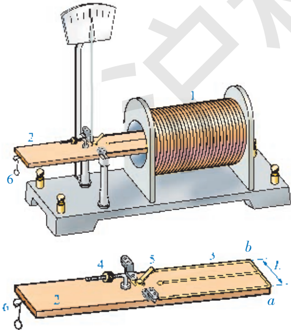
图 2-19 磁力秤
