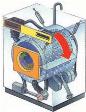
图 2-31 洗衣机甩干筒的壁上有许多小孔,当筒绕轴高速旋转时,衣物中的水从小孔中被甩出
