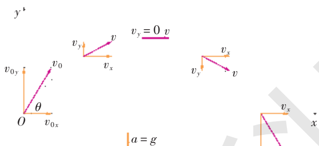
图 1-16 斜抛运动沿水平和竖直方向分解
