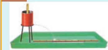
图 1-12 研究水柱的射程
