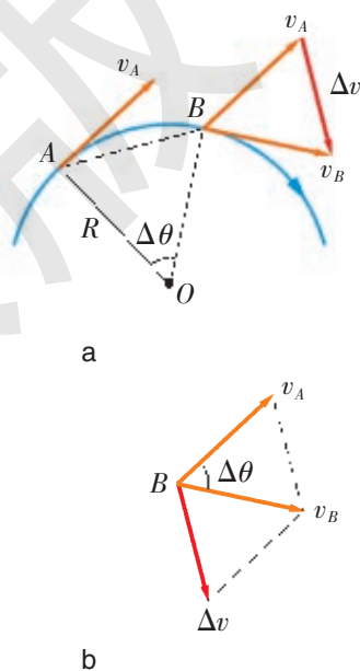
图 2-14 从速度合成的角度看圆周运动速度的变化
