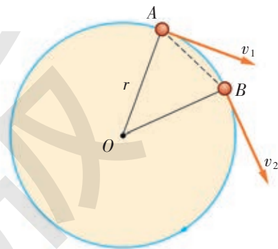
图 2-9 当 B 点无限逼近 A 点时, AB 之间的平均速度就是 A 点的瞬时速度
