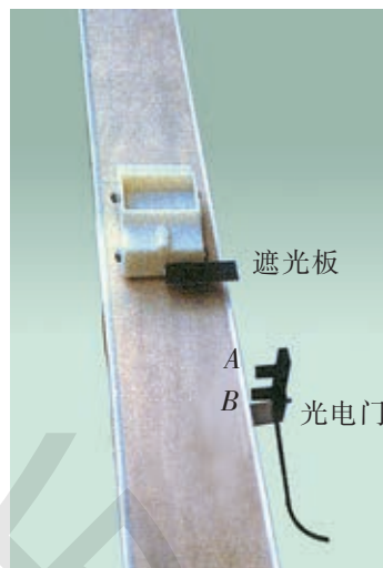
图 1-22 瞬时速度的测量
