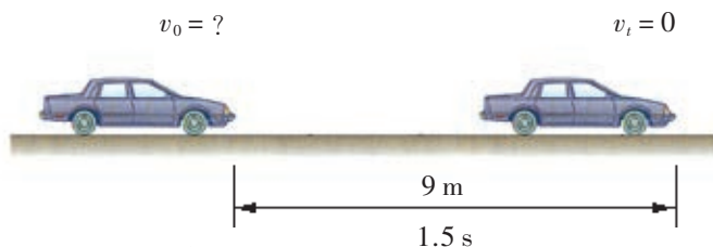
图 2-20 制动滑行
