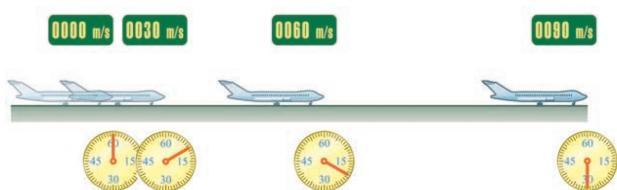
图 1-35 飞机匀加速滑行
