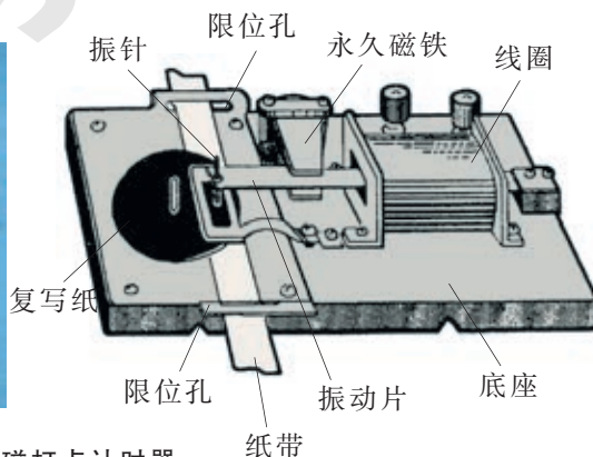
图 1-42 电磁打点计时器
