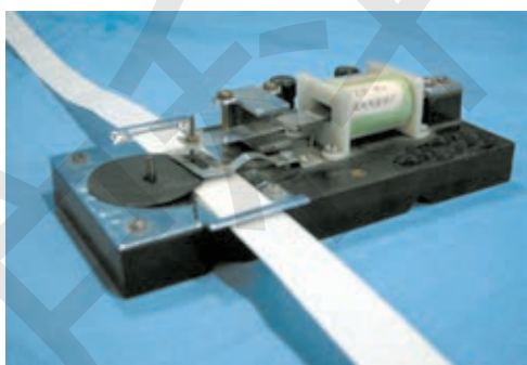
图 1-42 电磁打点计时器
