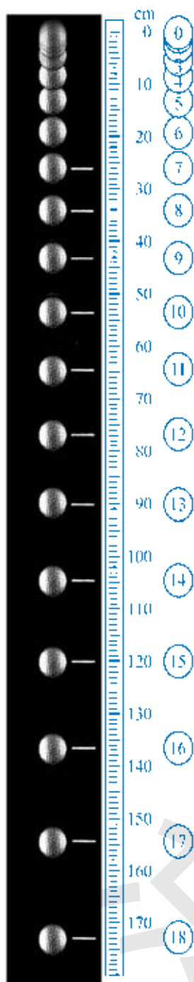
图 2-8 用频闪照相的方法拍摄的小球做自由落体运动的照片(两个像之间的时间间隔 \Delta t 为 0.033 s)
