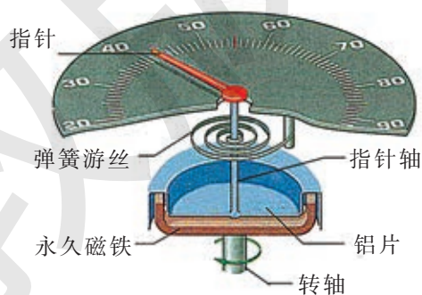
图 1-27 速率计的基本结构
