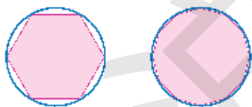
图 2-12 刘徽的“割圆术”
