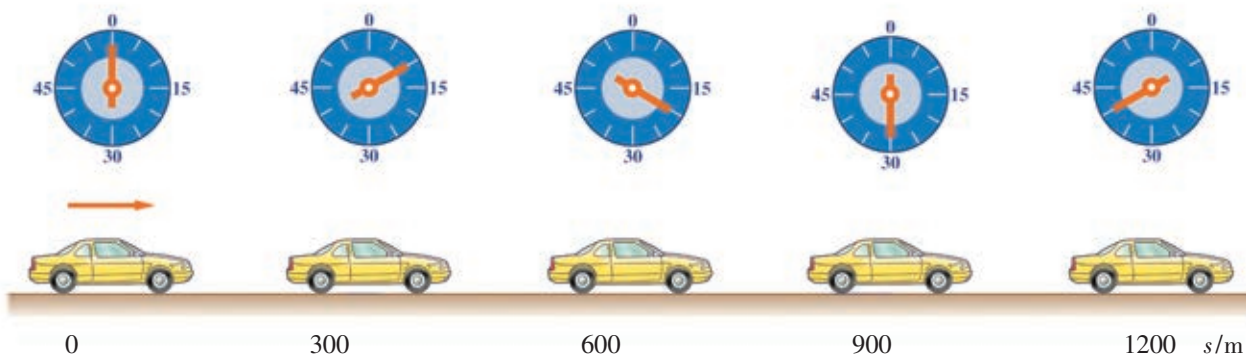
图 1-13 匀速直线运动
