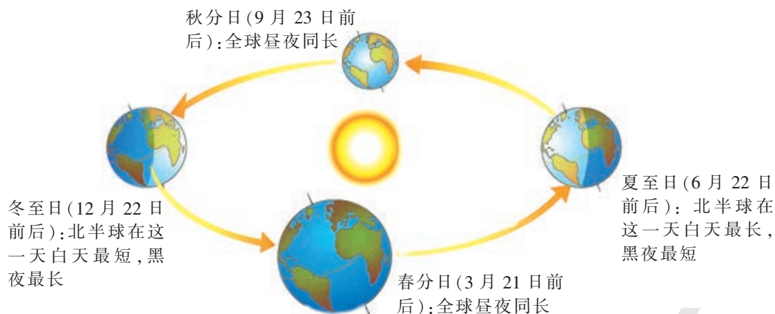
图 1-5 地球的公转和四季变化
