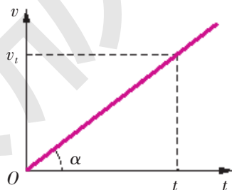
图 2-13 初速度为零的匀变速直线运动的 v-t 图像
